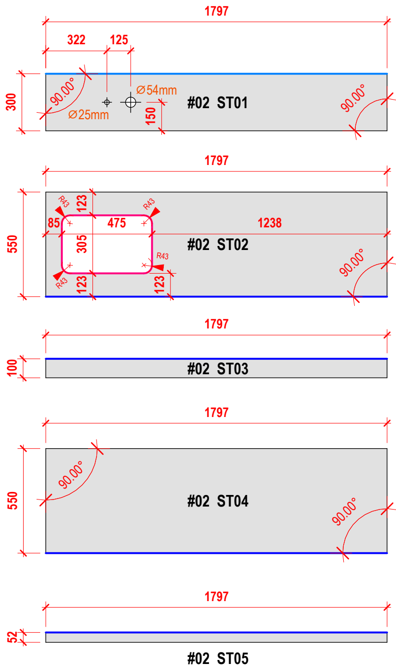
L1 BED 2 - PARTS 1 : 20
