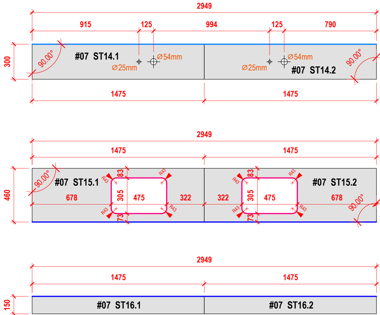
L1 MASTER ENSUITE - PARTS 1 : 20
